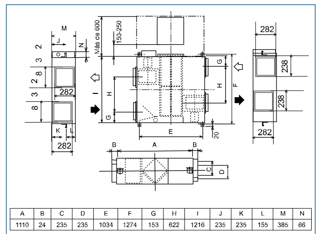
ERV0800ANN - ERV1000ANN
